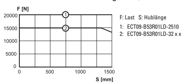
Verhältnis Knicklastgrenze / Hub
